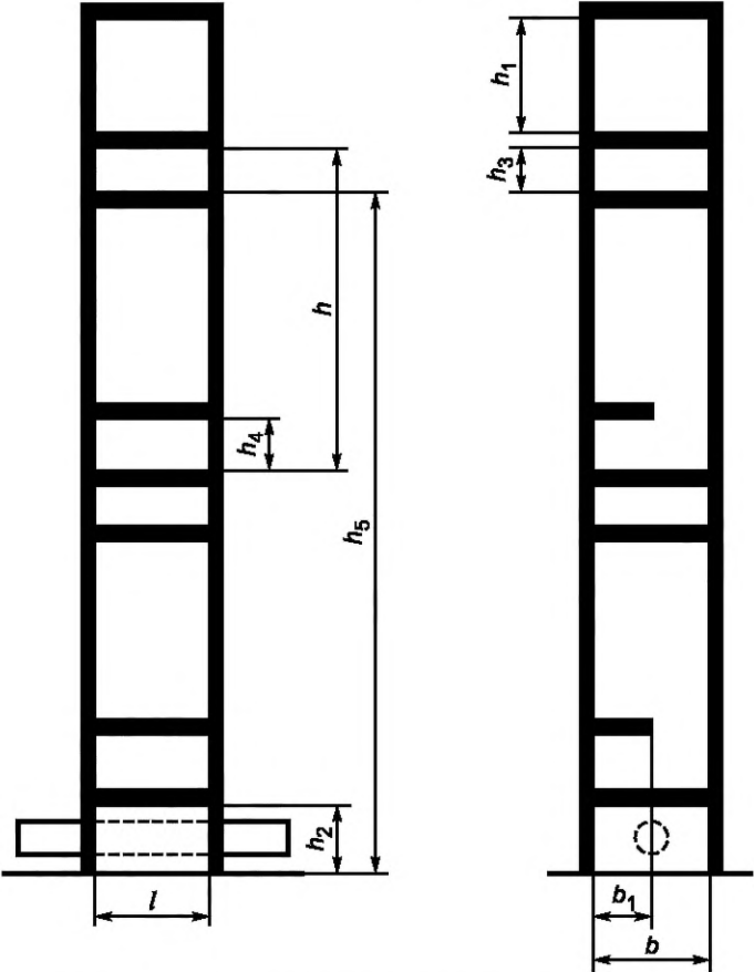
Рисунок 7 — Шкаф для детской одежды (до 3 лет включ.)
