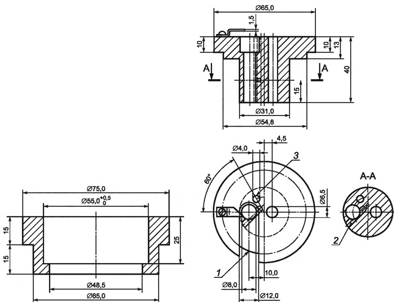
Рисунок 4 — Стопорное кольцо
