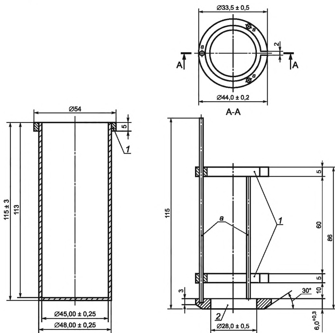
1 — серебряный припой
