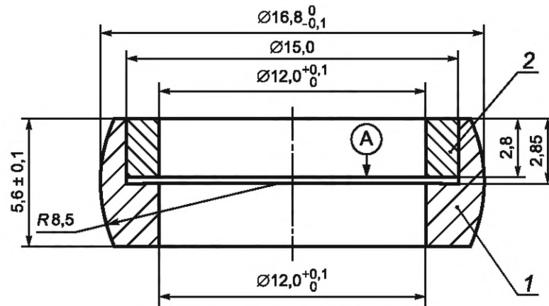
1 — держатель; 2 — стопорное кольцо
