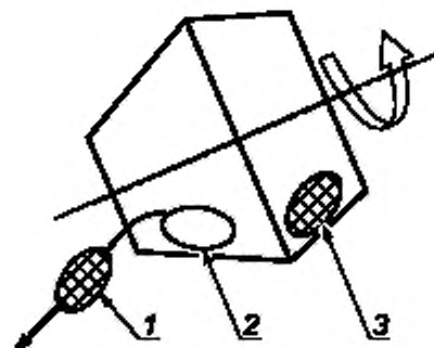
а) Определяющийся барабанный бетоносмеситель
