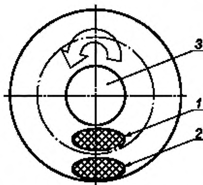
Рисунок 2 — Отбор проб из бетоносмесителя планетарного типа
