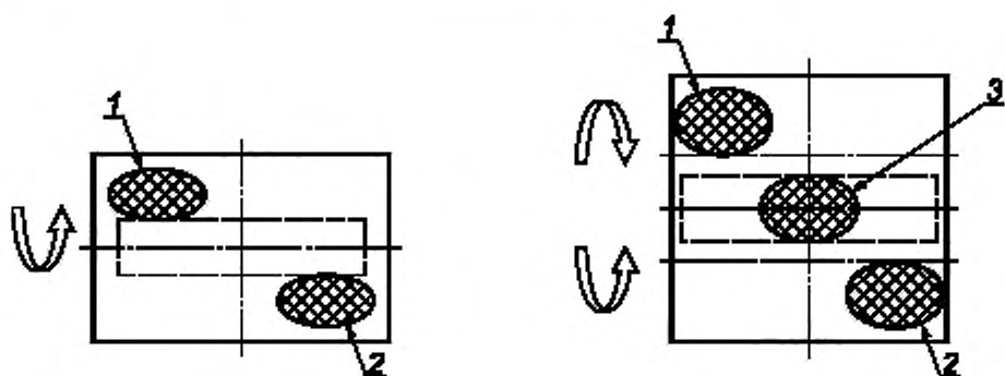
а) Одновалный бетоносмеситель
