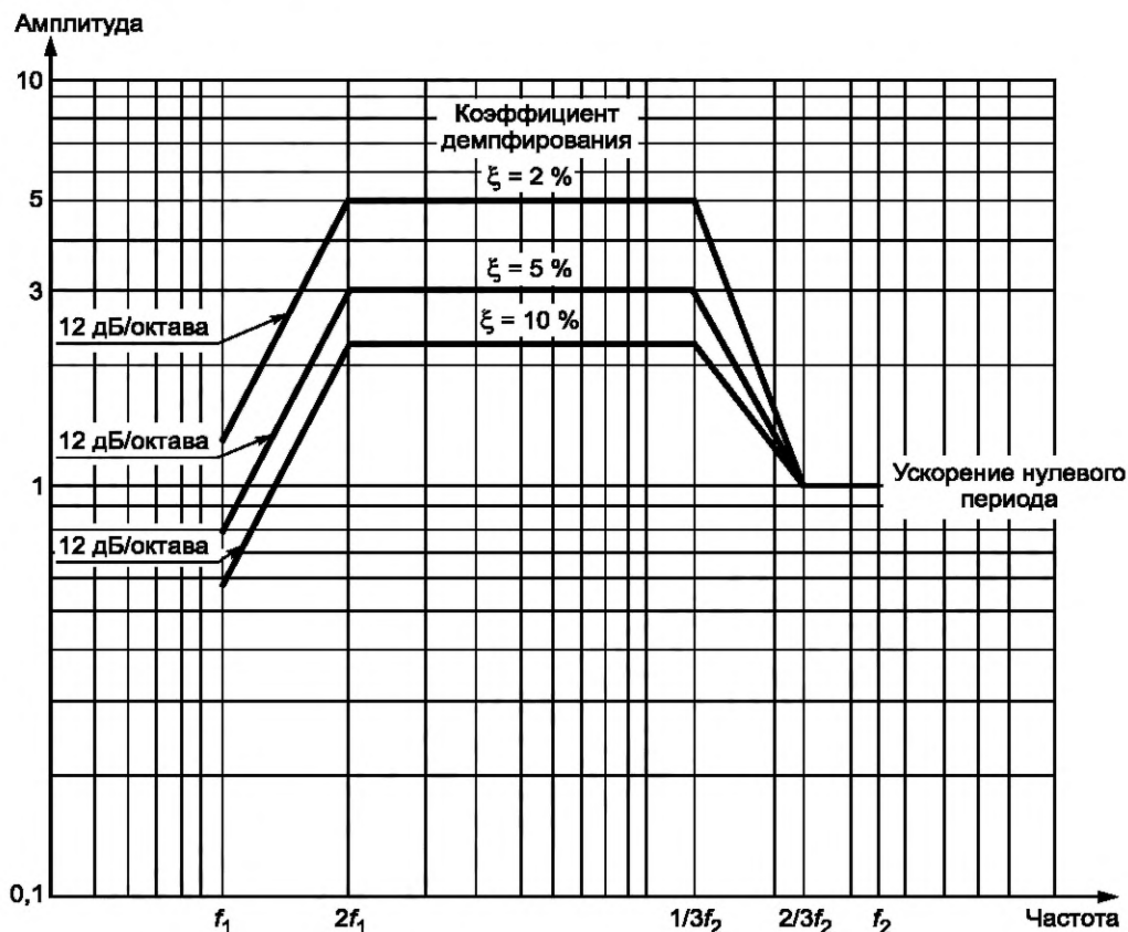
Рисунок A.1 — Рекомендуемая общая форма для заданного спектра отклика
