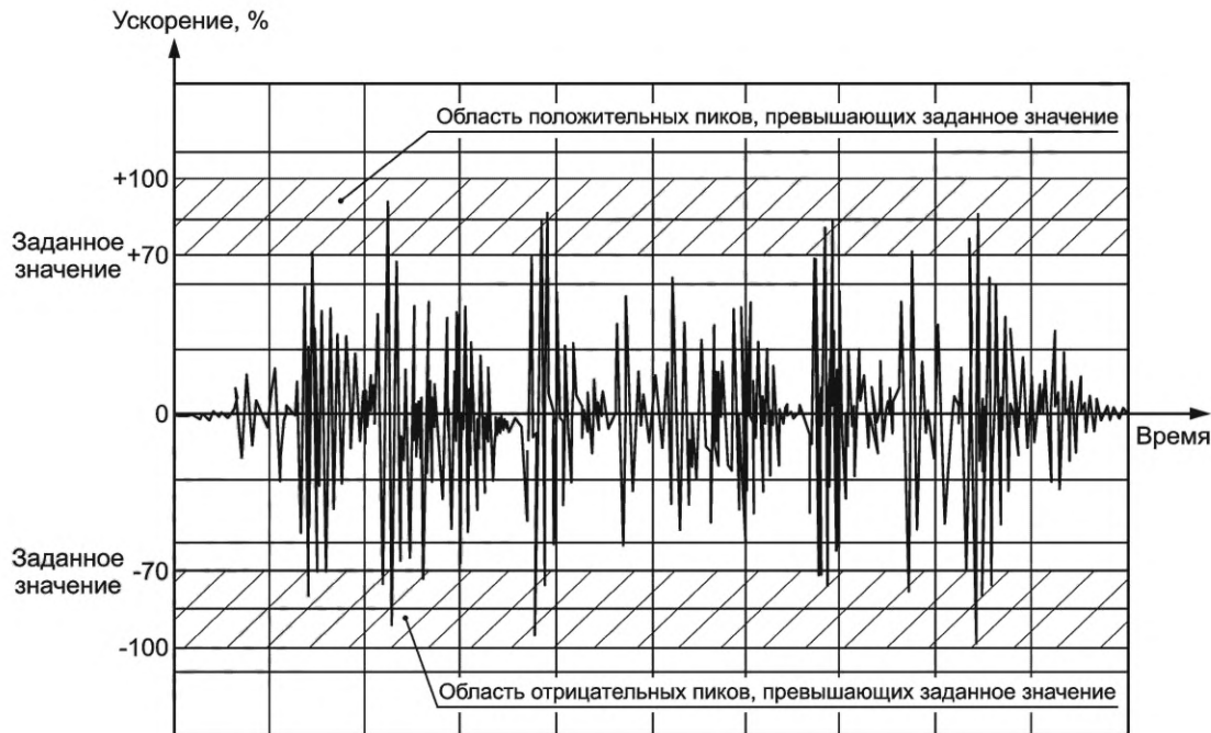
Рисунок 5 — Типичный отклик осциллятора на воспроизведенную акселерограмму процесса
