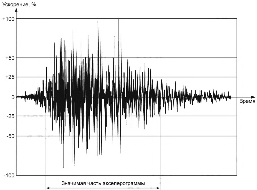
Рисунок 3 — Типичная форма акселерограммы
