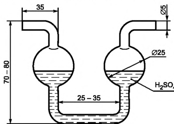
Рисунок 2 — Насадка
