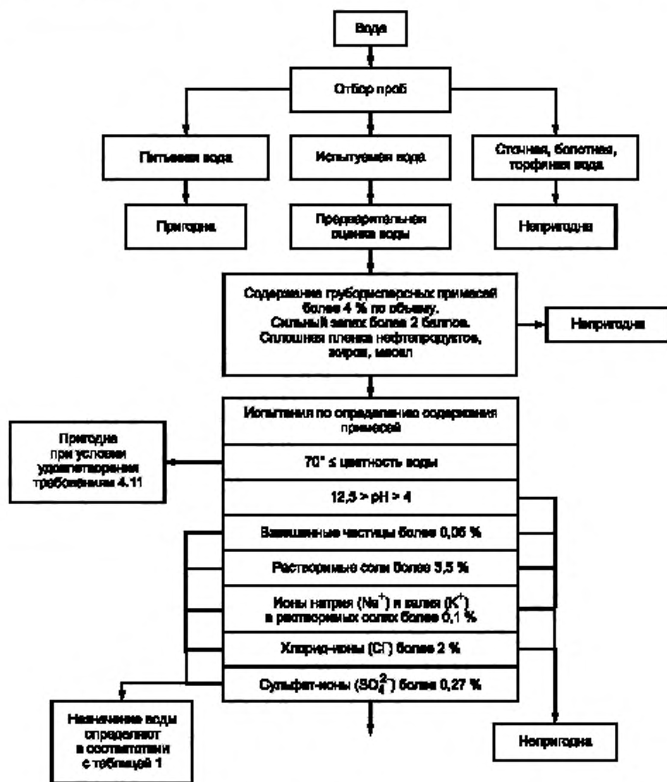
Рисунок Б.1, лист 1 — Схема проведения испытаний производственной воды для приготовления бетонов и строительных растворов
