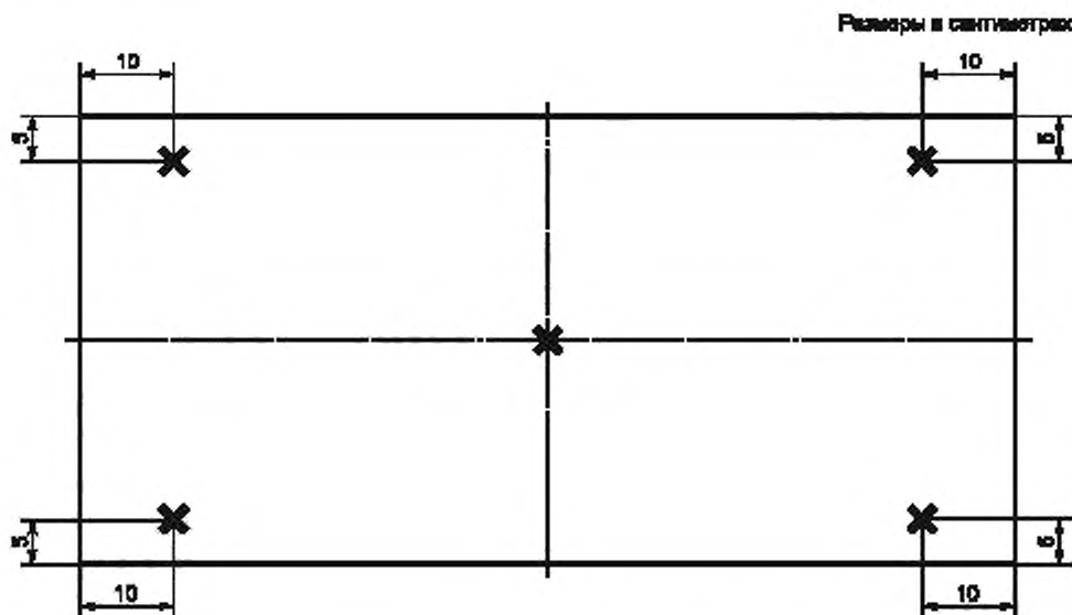
Рисунок G.1 — Положение термопары на верхней, средней и нижней проводной пластине
