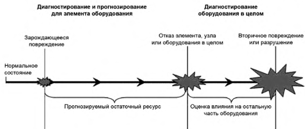
а) Развитие повреждения со временем
