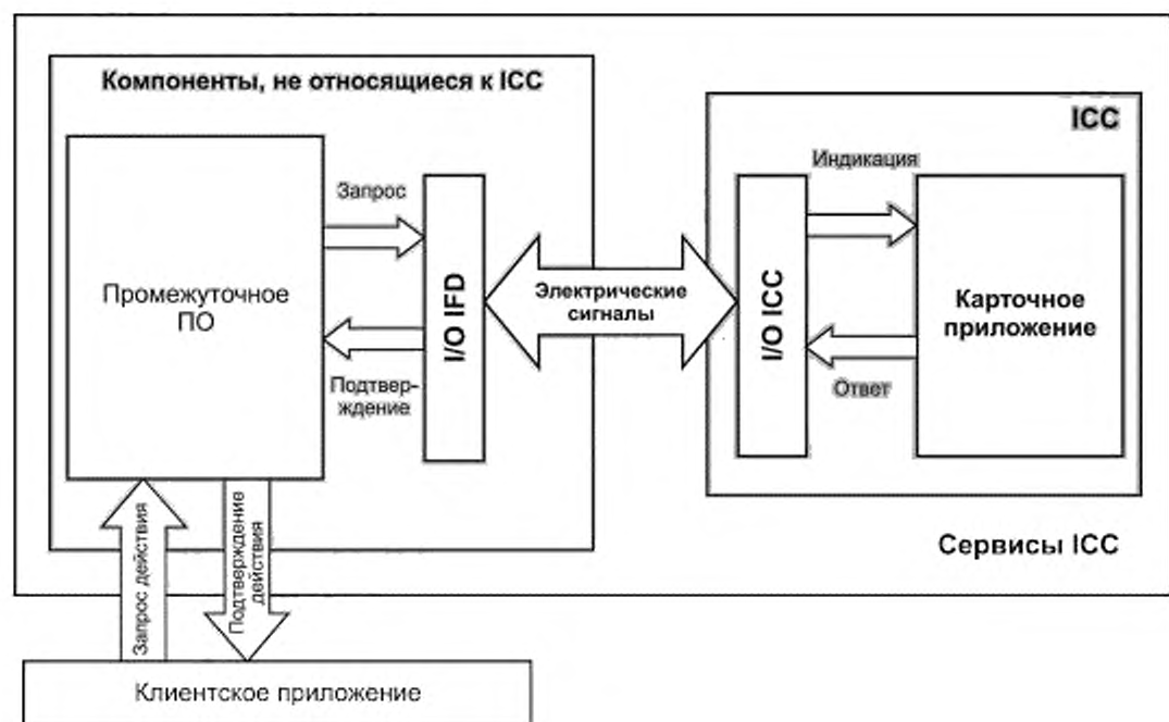
Рисунок А.1 — Физическая архитектура
