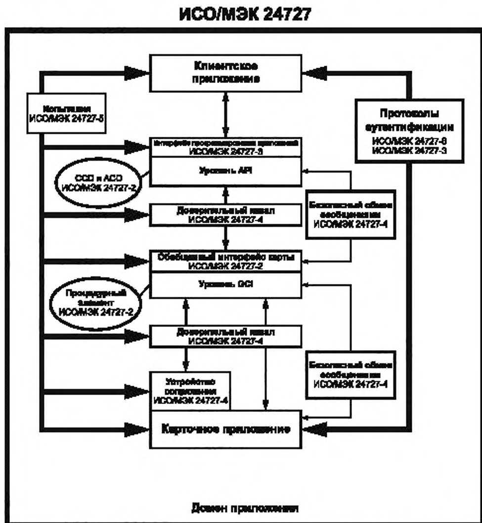
Рисунок 1 — Логическая архитектура по стандартам серии ИСО/МЭК 24727
