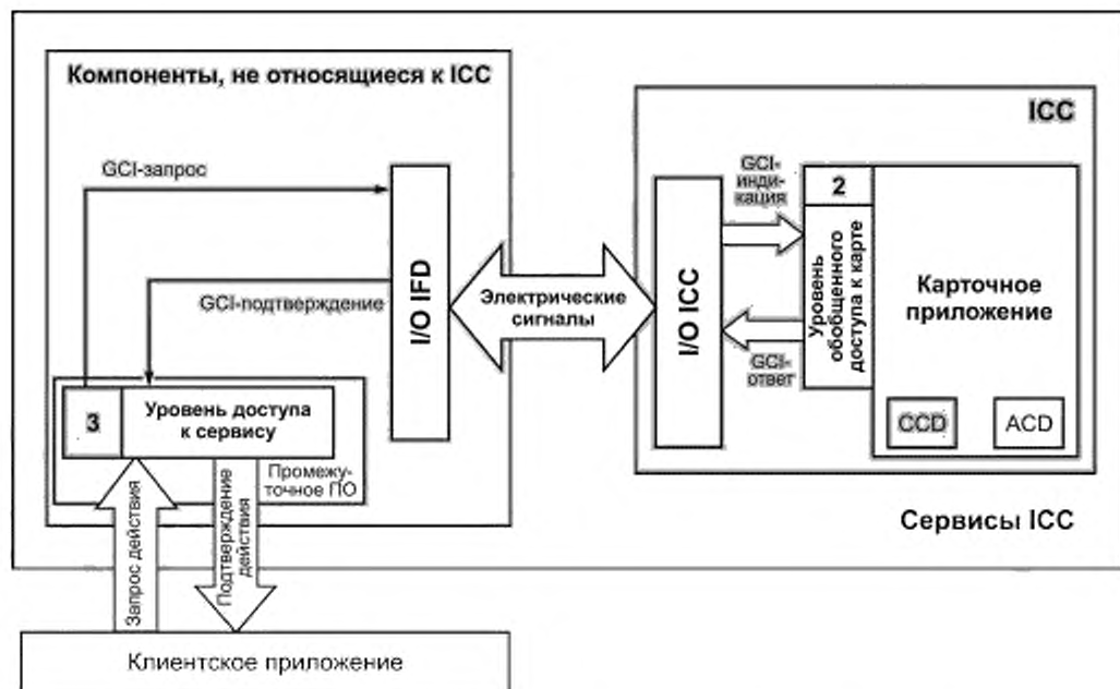
Рисунок А.4 — Уровень обобщенного доступа к карте, реализованный на ICC
