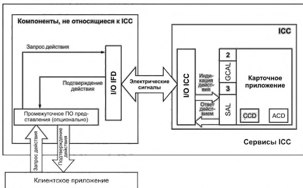
Рисунок А.5 — Уровни доступа к сервису и обобщенного доступа к карте, реализованные на ICC
