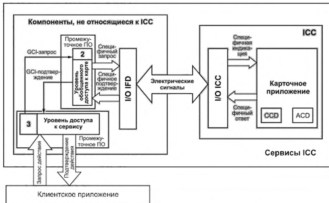
Рисунок A.2 — Отдельная реализация каждого интерфейса и уровня
