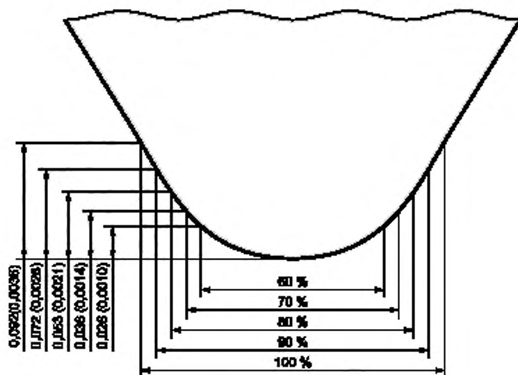
Рисунок Е.3 — Пример стилиуса с углом 60^\circ и радиусом 0,102 мм (0,004 дюйма)
