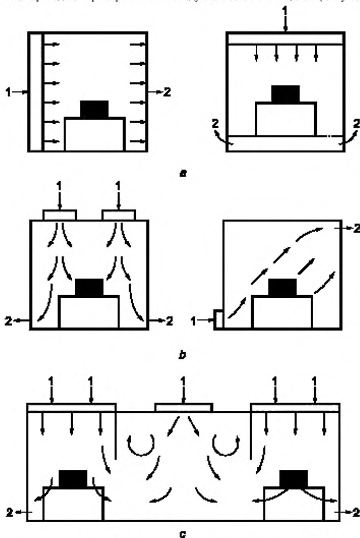
а — одинаправленный поток воздуха; б — неодинаправленный поток воздуха; в — смешанный поток воздуха; 1 — приточный воздух; 2 — вытяжной воздух
