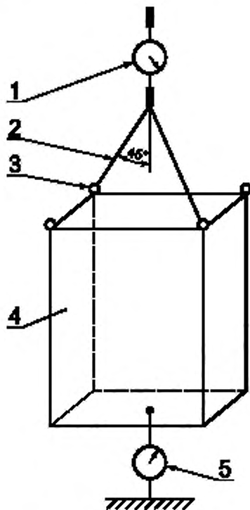
1 — динамометр; 2 — строп; 3 — строповое устройство; 4 — ВРУ; 5 — динамометр 2
