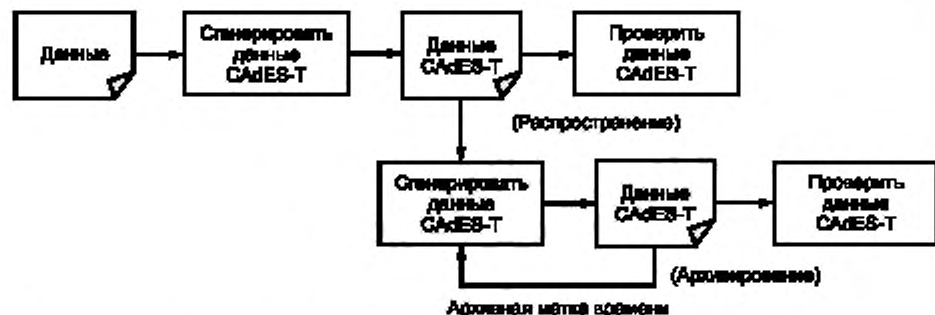
Рисунок 7 — Отношения между данными, соответствующими спецификациям CAAdES-T и CAAdES-A
