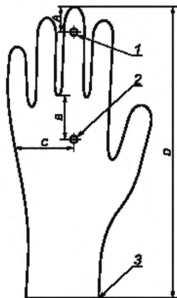
Рисунок 1 — Расположение точек измерения толщины перчатки
