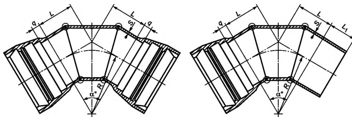
а) Отвод раструбный (ОР)
