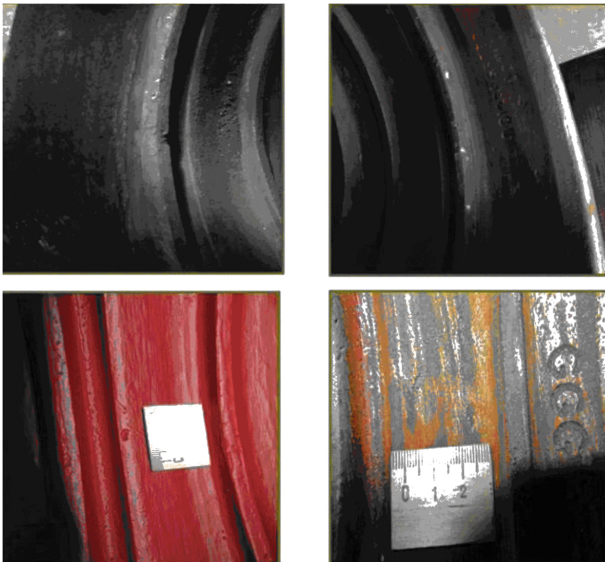
Рисунок Д.5 — Засор
