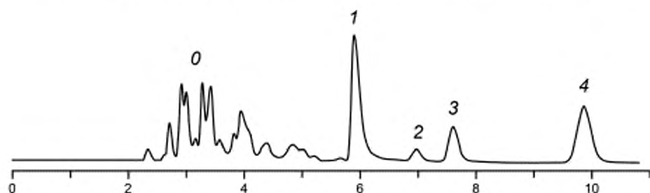
0 — матрица; 1 — этанол; 2 — бензол 1 %, 3 — втор-бутиловый спирт; 4 — толуол
