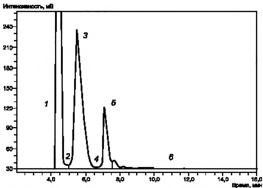
Рисунок 1 — Пример хроматограммы образца авиационного топлива с указанием точек начала и конца интегрирования и типов ароматических соединений
