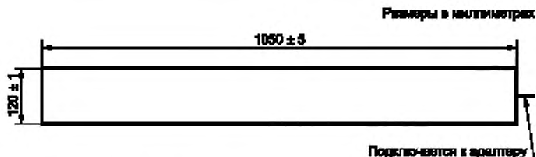
Рисунок 7 — Преобразовательная пластина для калибровки клещей связи
