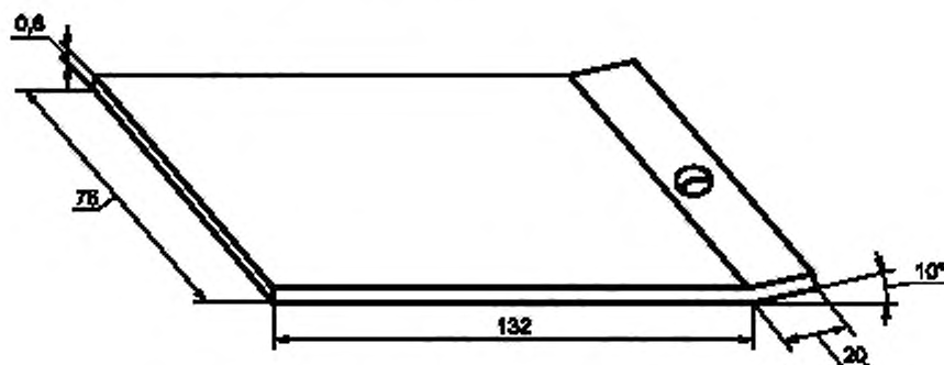
Рисунок 2 — Испытательная металлическая пластина
