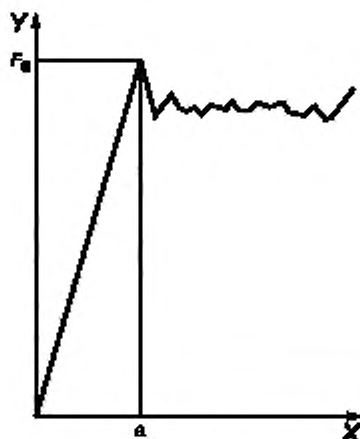
Рисунок 4 — Типичный пример записанного графика F_s , имеющего пик
