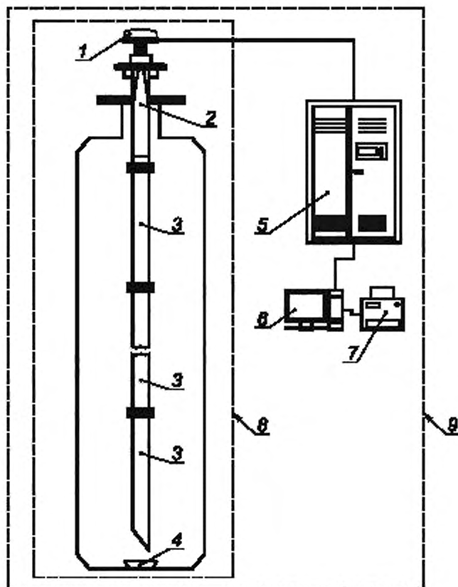
1 — микроволновой передатчик; 2 — антенна; 3 — стальная трубка; 4 — аттенуатор; 5 — управляющий блок; 6 — дисплейный блок; 7 — принтер; 8 — АРУ; 9 — система АРУ
