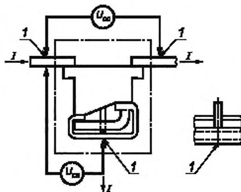
1 — места измерения падения напряжения
