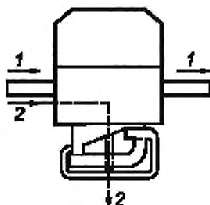
Рисунок 5 — Схема испытания на тепловой кратковременно выдерживаемый ток
