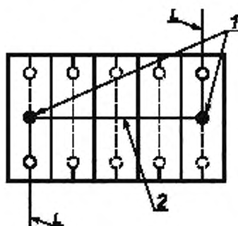
1 — место измерения превышения температуры; 2 — рейка крепления колодки; L — проводники длиной 1 м
