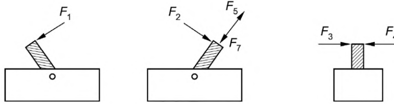
Рисунок 3b — Рычаг
