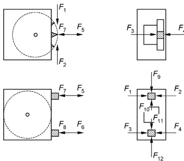
Рисунок 3e — Диск
