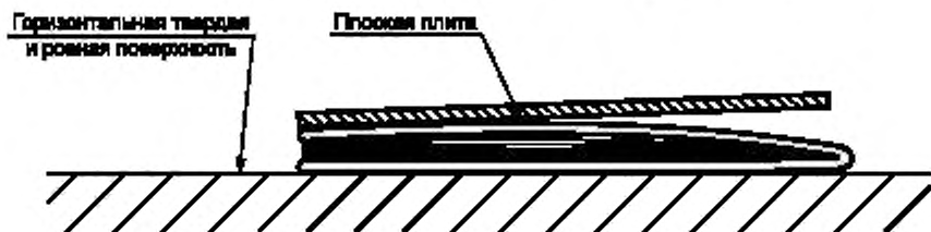
Рисунок 19 — Расположение MRP при измерении коробления
