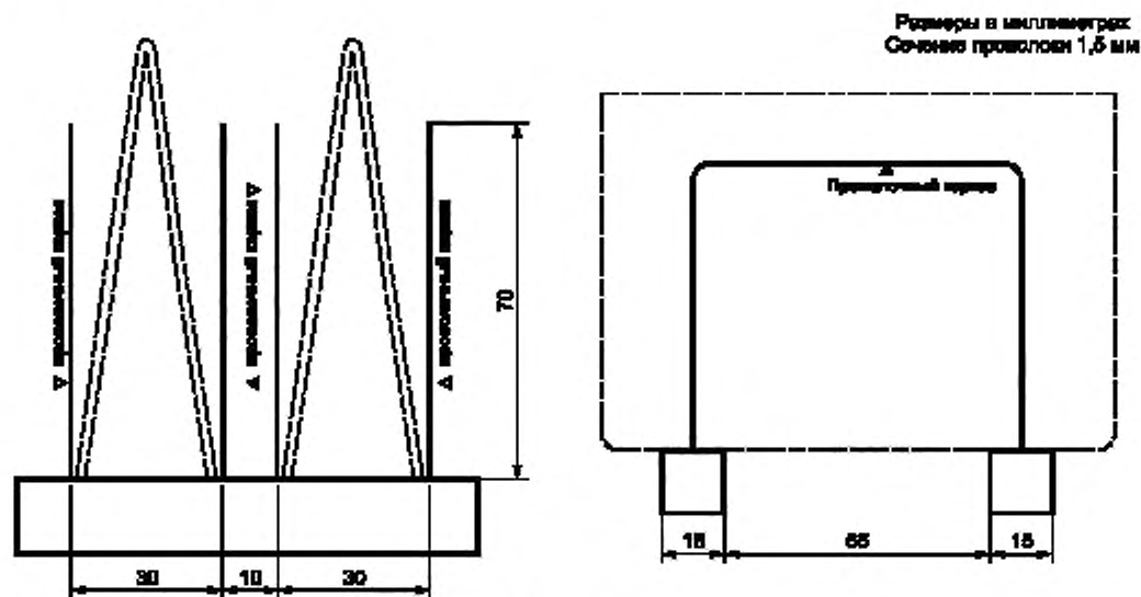
Рисунок 2 — Держатель MRP
