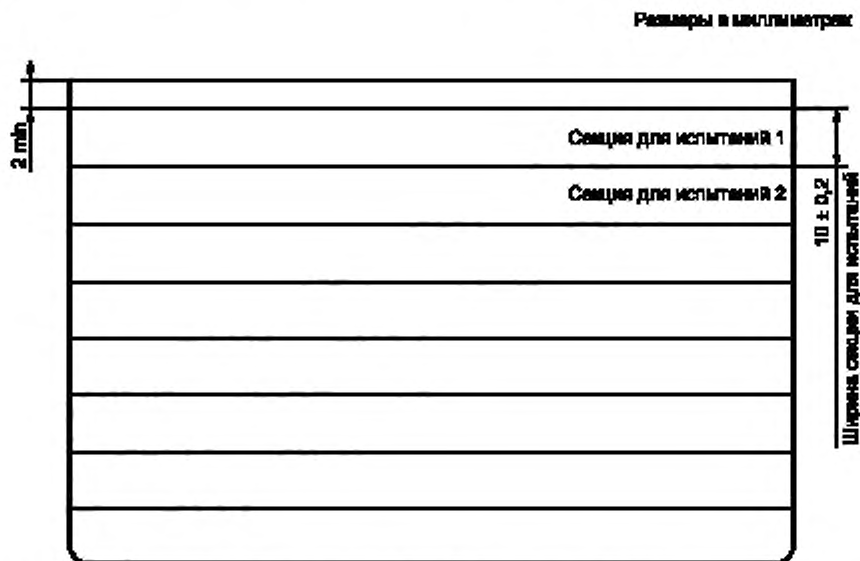
Рисунок 16 — Подготовка образца к измерению прочности сцепления
