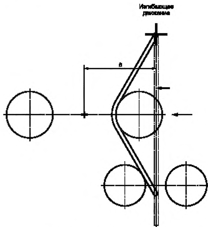
Рисунок 10 — Изгибающее движение
