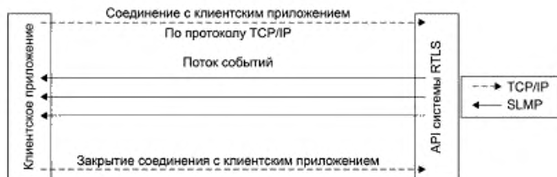
Рисунок 1 — Архитектура протокола SLMP
