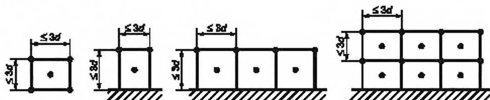
Рисунок ДА.1 — Схема определения точек измерения, когда ребро измерительной поверхности превышает 3 м
