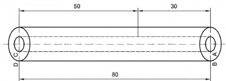
Рисунок В.1 — Форма и размеры образца
