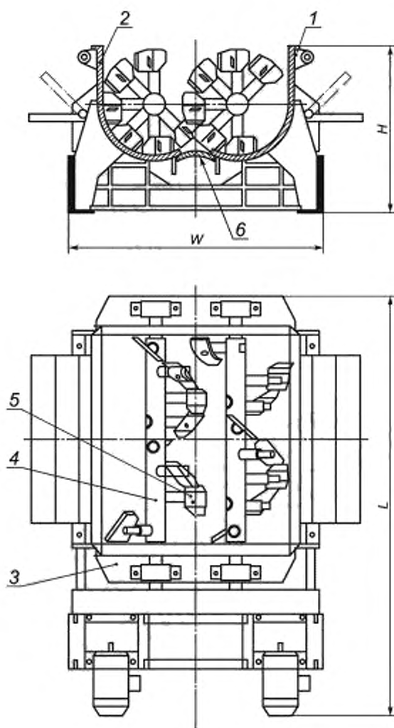
Рисунок А.12 — Двухвальный лопастной бетоносмеситель
