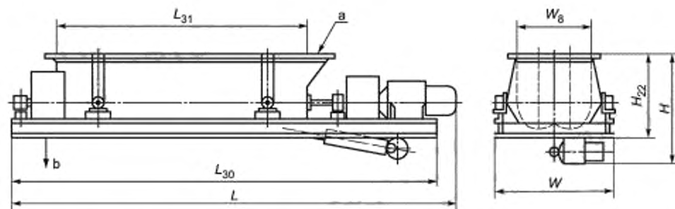
Рисунок А.14 — Лопастной бетоносмеситель со скиповым подъемником, расположенным на опорной конструкции
