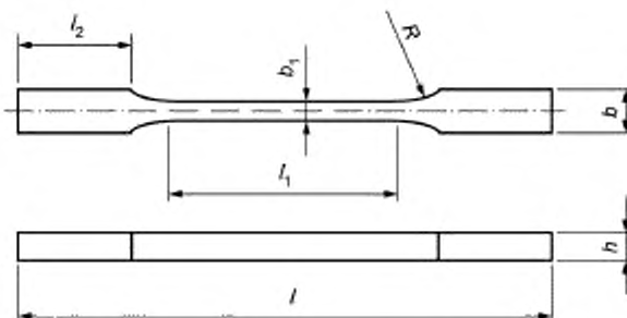
l — длина образца; l_1 — длина рабочей части образца; l_2 — длина захвата; b — ширина образца; b_1 — ширина рабочей части образца; h — толщина образца; R — радиус закругления
