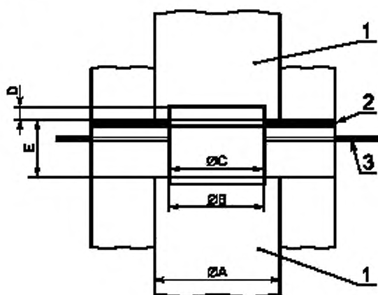
1 – микрофон; 2 – изолятор; 3 – капиллярные трубки
