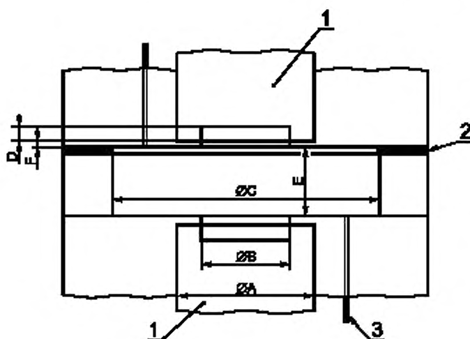
1 — микрофон; 2 — изолятор; 3 — капиллярные трубки
