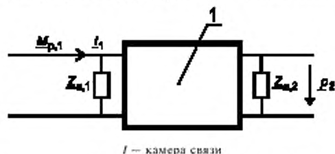
Рисунок 1 — Эквивалентная схема для определения акустического передаточного импеданса \underline{Z}_{a,12}
