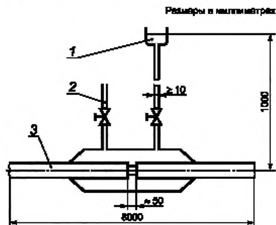
1 — резервуар с водой; 2 — вентиляционное отверстие; 3 — кабель
