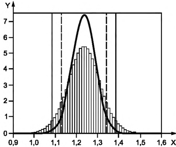
Рисунок 10 — Аппроксимации плотности распределения вероятностей для выходной величины \delta m , полученные с использованием способа оценивания неопределенности по GUM с учетом членов первого порядка и методом Монте-Карло
