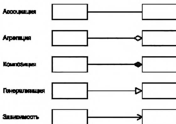
Рисунок 1 — Символика UML
