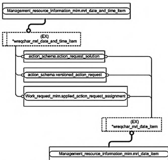
Рисунок D.4 — Представление IMM на уровне объектов в формате EXPRESS-G. Диаграмма 3 из 5
