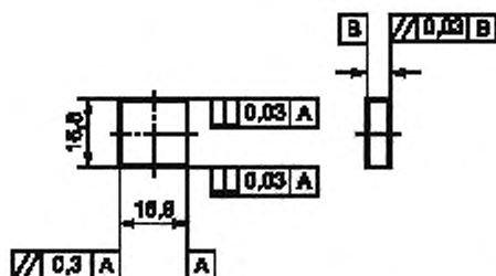
Рисунок 7 — Образец квадратного сечения
