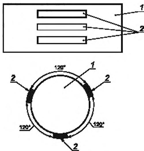
1 — образец; 2 — тензорезистор
