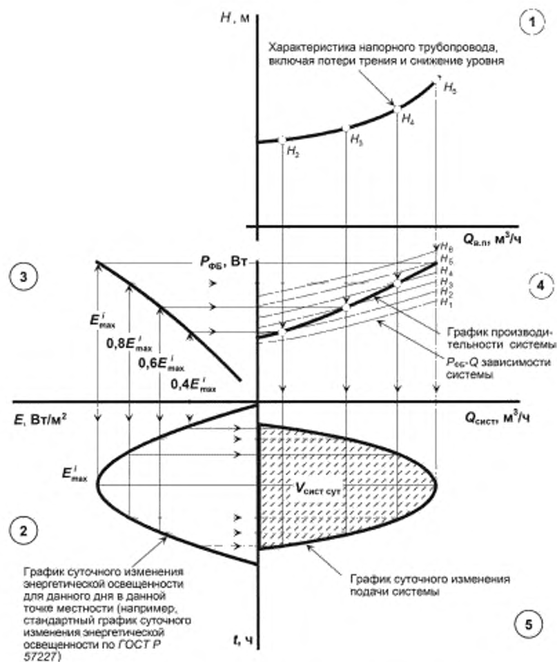
Рисунок 4 — Пример номограммы выходных характеристик автономной фотоэлектрической насосной системы для подачи воды (система с центробежным насосом, тип А)
