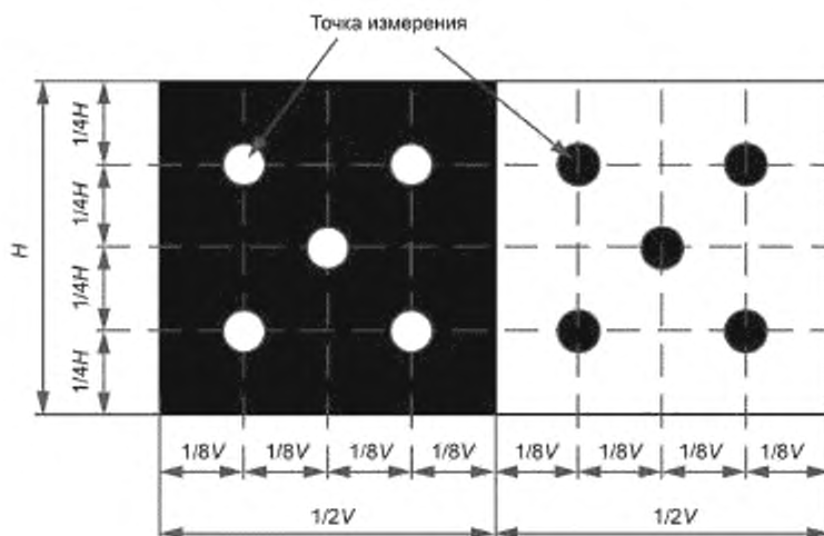
Рисунок 3 — Точки измерения
