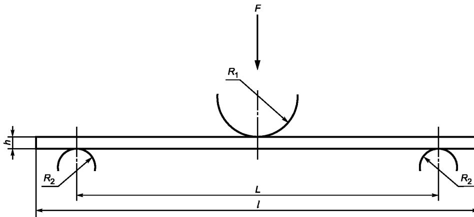
Рисунок 2 — Схема трехточечного нагружения
