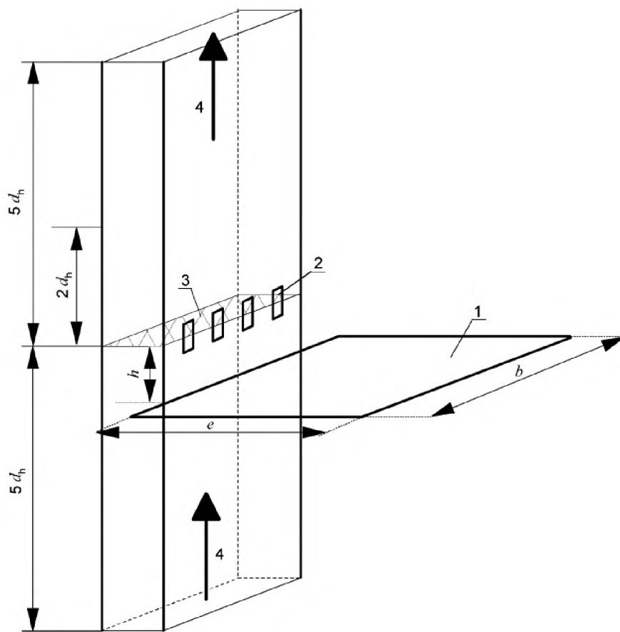
1 — рабочая платформа; 2 — измерительный порт; 3 — измерительная плоскость; 4 — направление движения потока; b — длина рабочей зоны; d_h — гидравлический диаметр газохода; e — ширина рабочей зоны; h — минимальная высота свободной зоны над рабочей платформой
