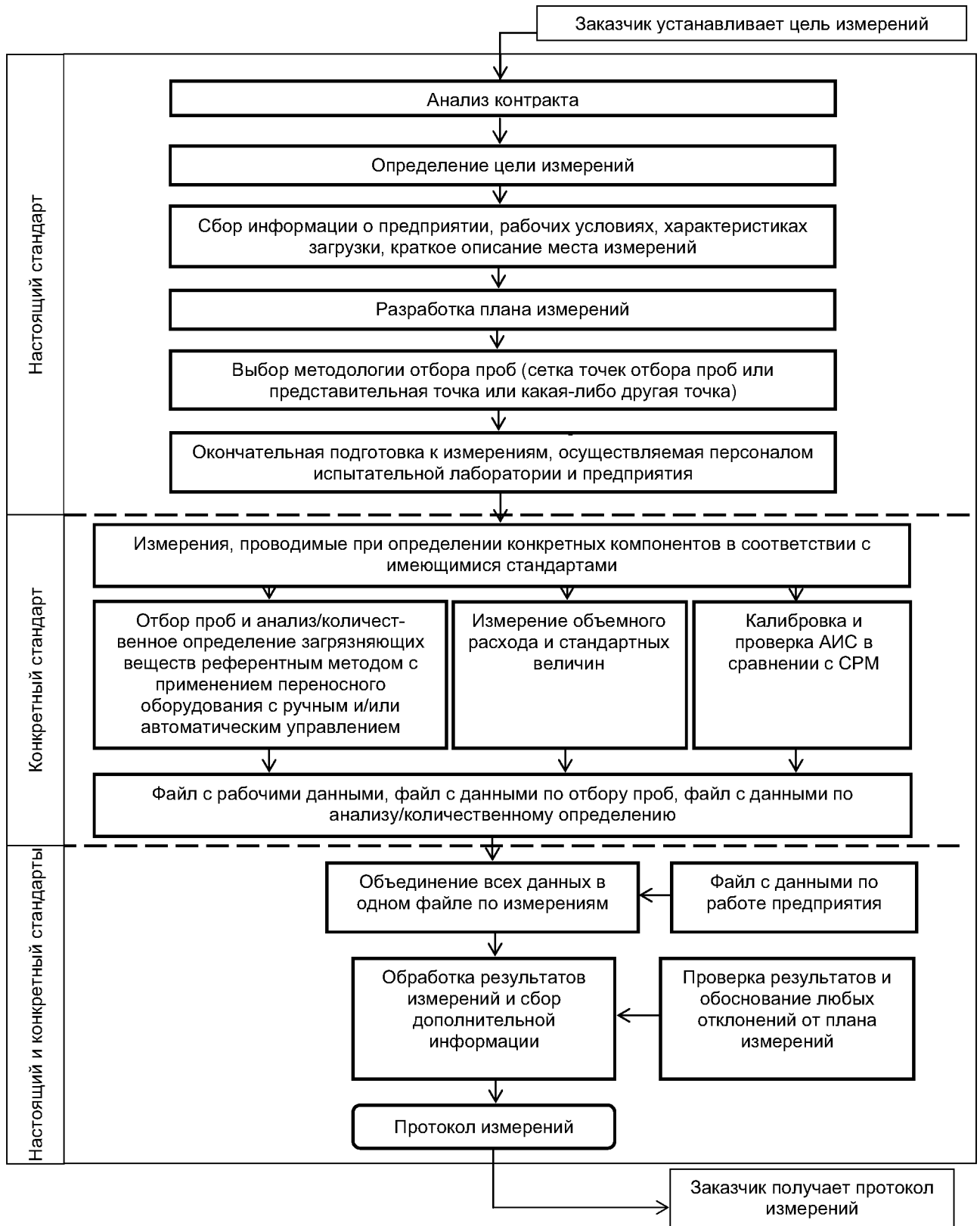
Рисунок 1 — Основные этапы периодических измерений выбросов стационарных источников
