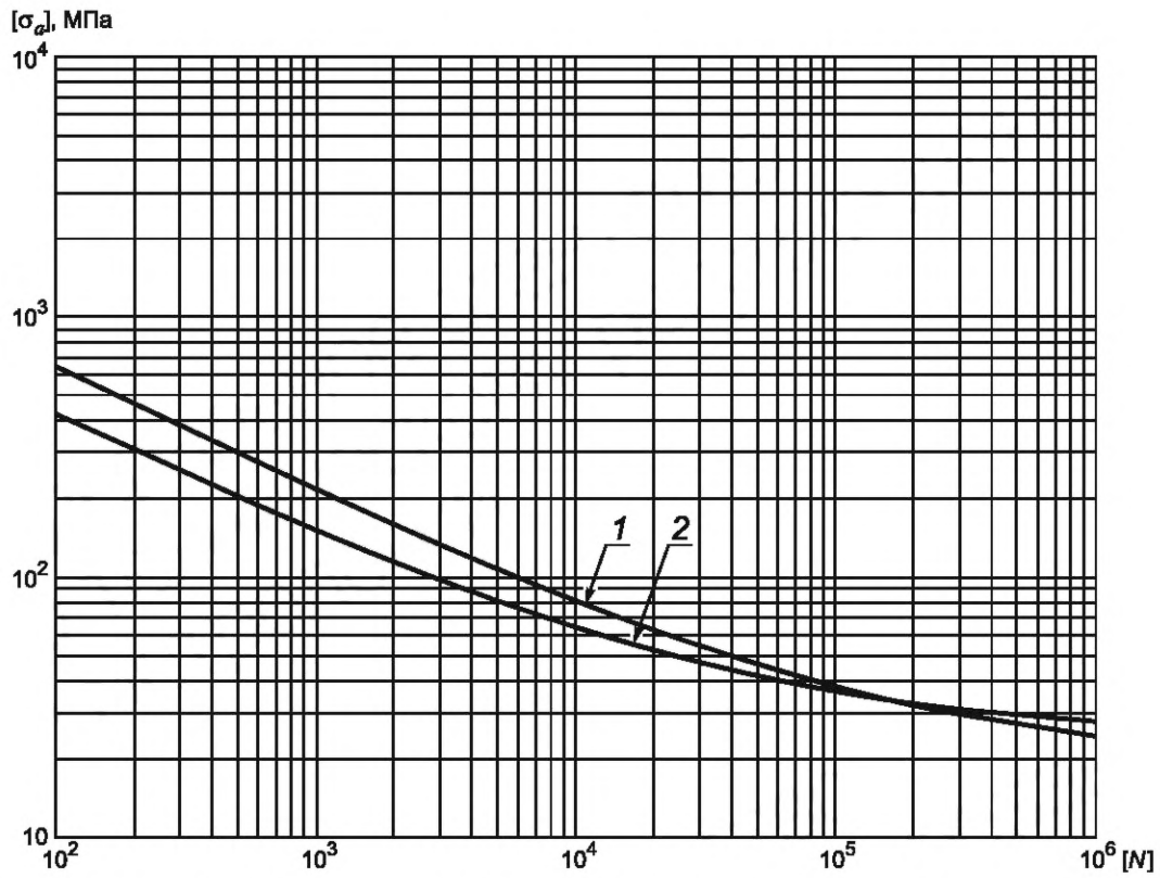
Рисунок 8 — Расчетная кривая усталости для сплавов титана
