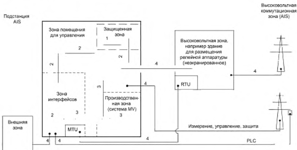
MTU — основное оконечное устройство; RTU — удаленное оконечное устройство; PLC — связь по силовым линиям
