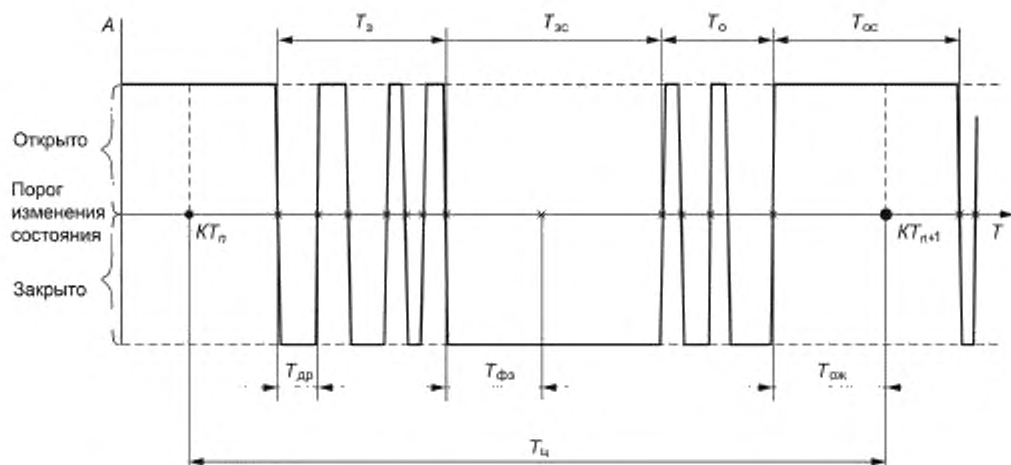
Рисунок 4 — Цикл управляющего сигнала при испытании счетчика на ложные срабатывания
