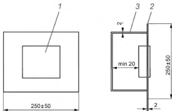
1 — счетчик, 2 — стальная установочная плита; 3 — стальная крышка
