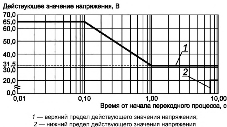
Рисунок 11 — Пределы приведенных значений ненормальных повышенных и пониженных напряжений первичных систем постоянного тока 27 В
