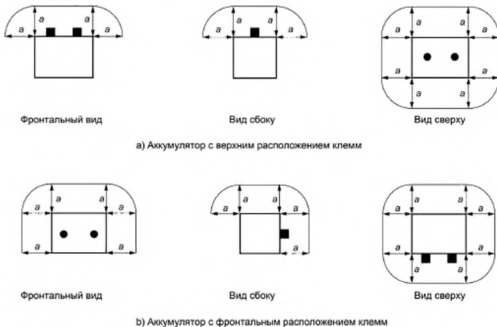
Рисунок 1 — Свободное пространство a вокруг аккумулятора
