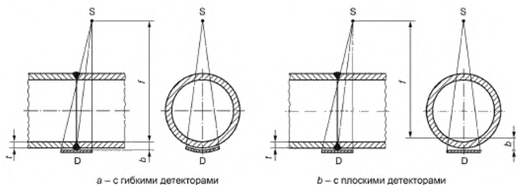
Рисунок 13 — Схема контроля изогнутых объектов при просвечивании через две стенки (одно изображение) для контроля стенки, ближайшей к детектору: IQI располагается на детекторе
