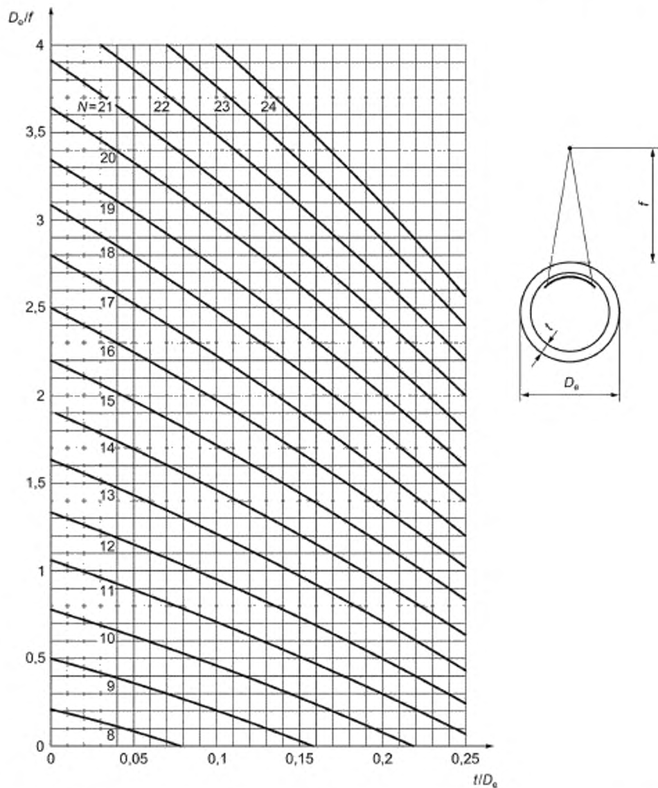
Рисунок А.1 — Минимальное количество экспозиций N при просвечивании через одну стенку с источником излучения снаружи, при максимально допустимом увеличении просвечиваемой толщины \Delta t из-за наклонного направления излучения в проверяемой области, равном 10 % (класс В), как функция отношений t/D_e и D_e/f
