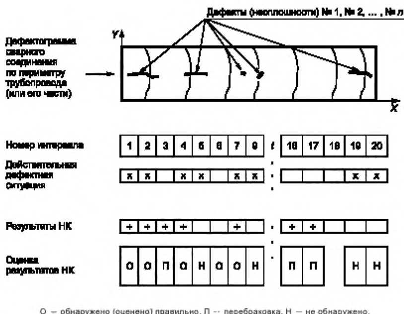
Рисунок Е.1 — Пример процедуры сравнения результатов НК с действительной дефектной ситуацией для расчета показателей достоверности результатов контроля
