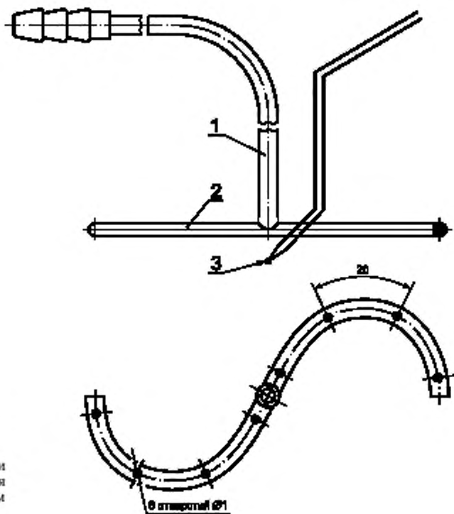
Рисунок И.4 — Устройство для отбора проб и измерения температуры продуктов сгорания для дымохода диаметром, не превышающим 100 мм
