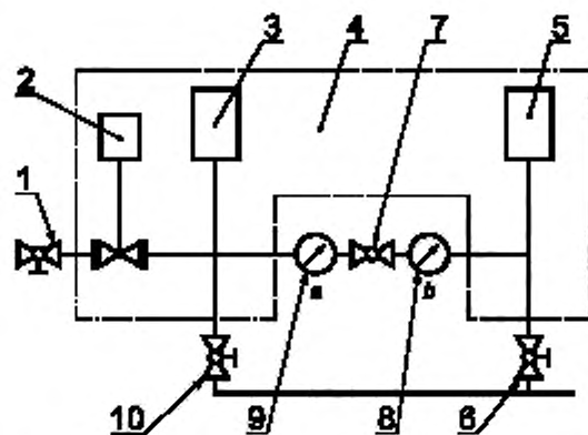
Рисунок И.7 — Проверка герметичности компонентов газового тракта (метод потери давления)
