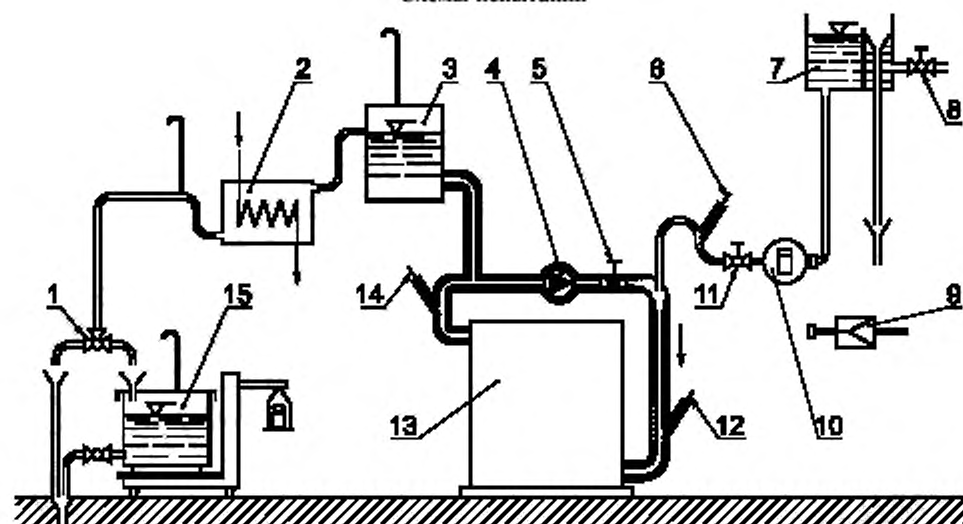
Рисунок И.1 — Испытательный стенд с прямой рециркуляцией
