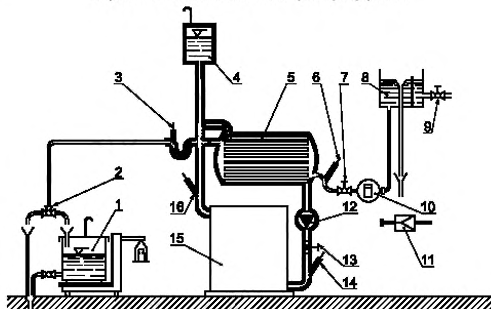
Рисунок И.1 — Испытательный стенд с прямой рециркуляцией
