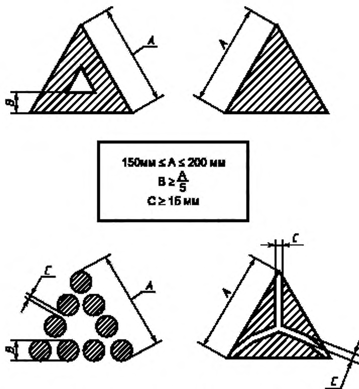
Рисунок 1 — Отражатели света для прицепов класса III A
