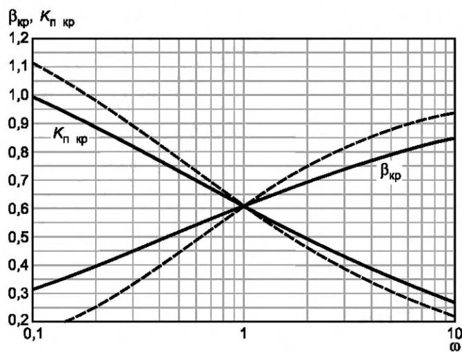
Рисунок Е.3 — Коэффициенты \beta_{кр} и K_{п\ кр} для омега-метода
