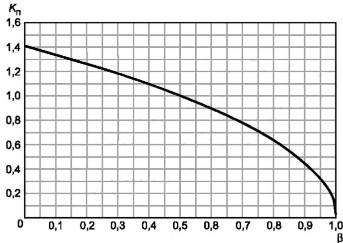
Рисунок Е.1 — Коэффициент K_n для несжимаемой жидкости
