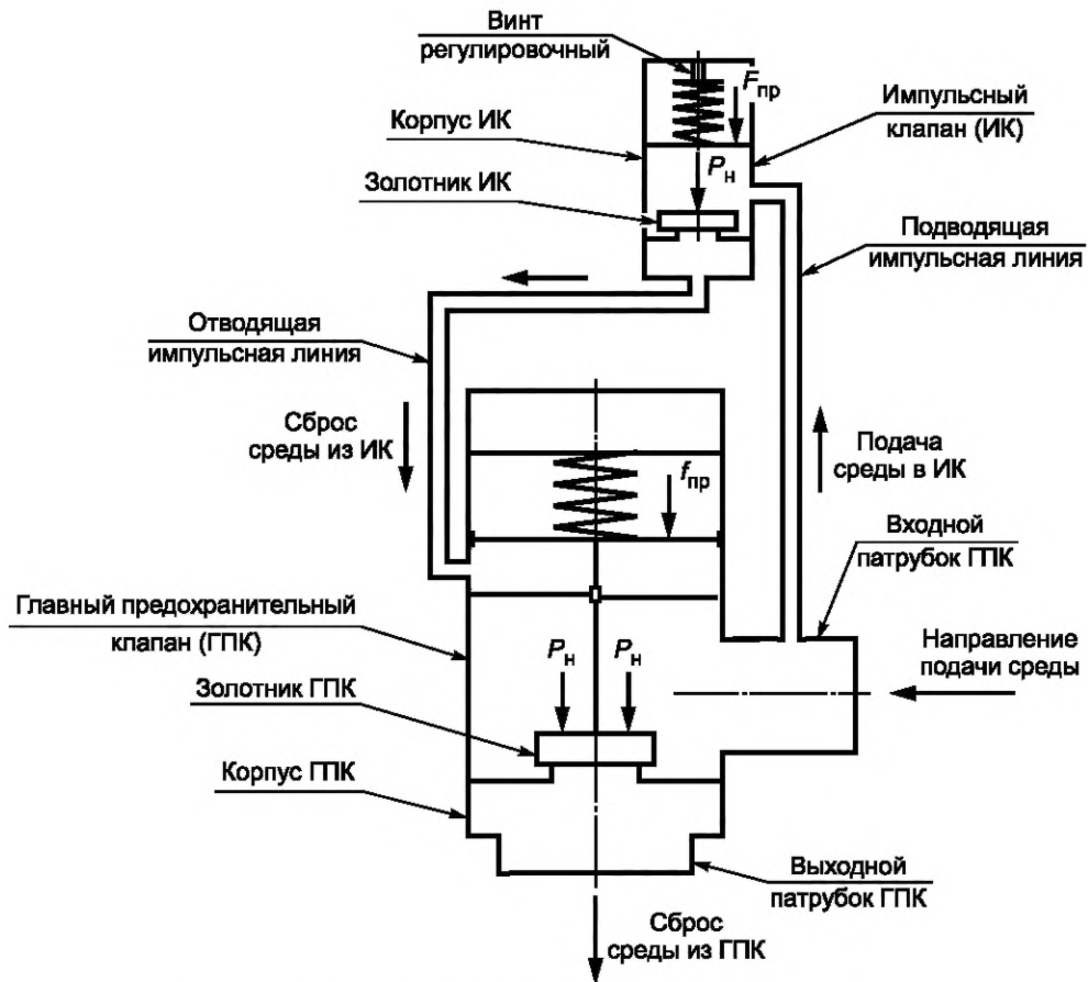
Рисунок В.3 — Импульсно-предохранительное устройство
