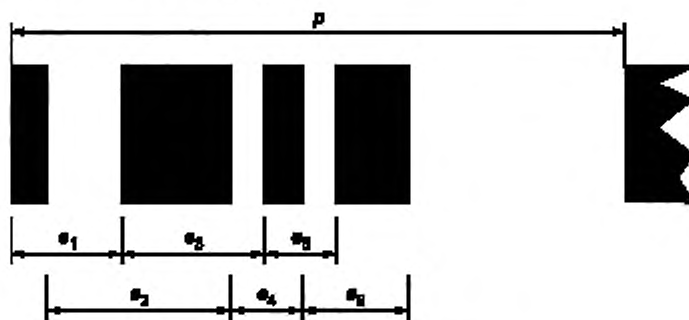
Рисунок J.1 — Размеры для декодирования
