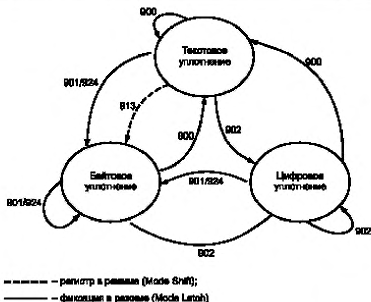
Рисунок 5 — Возможные переходы между режимами
