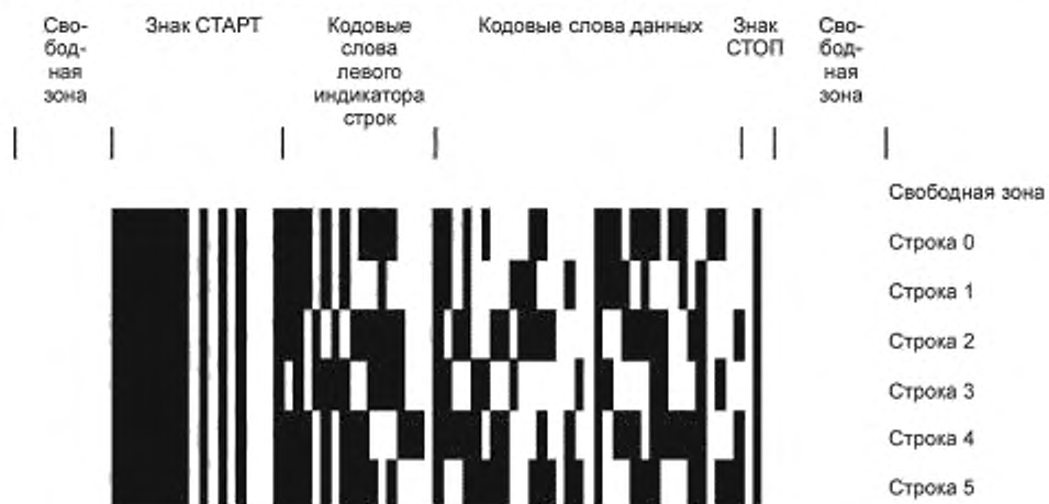
Рисунок G.1 — Компакт PDF417
