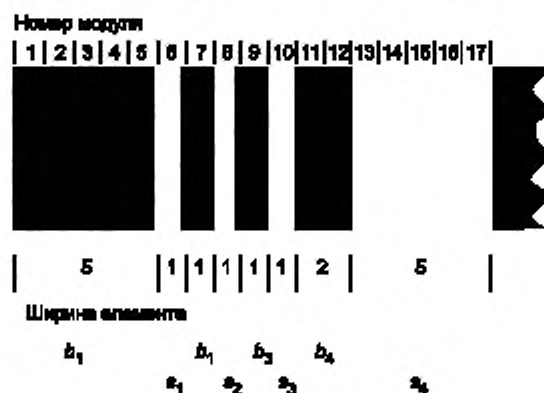
Рисунок 3 — Знак символа PDF417
