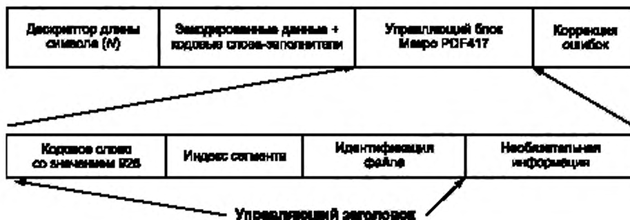
Рисунок Н.1 — Схемы символов PDF417
