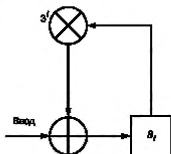
Рисунок К.1 — Делитель синдрома символа
