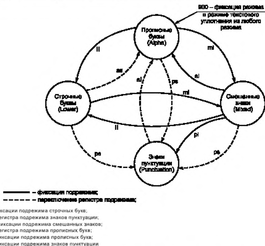
Рисунок 6 — Переключения подрежимов в режиме текстового уплотнения
